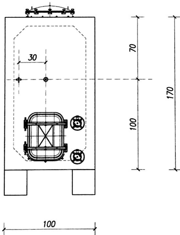
N°9 CISTERNE CON CAPACITA' 25hl
