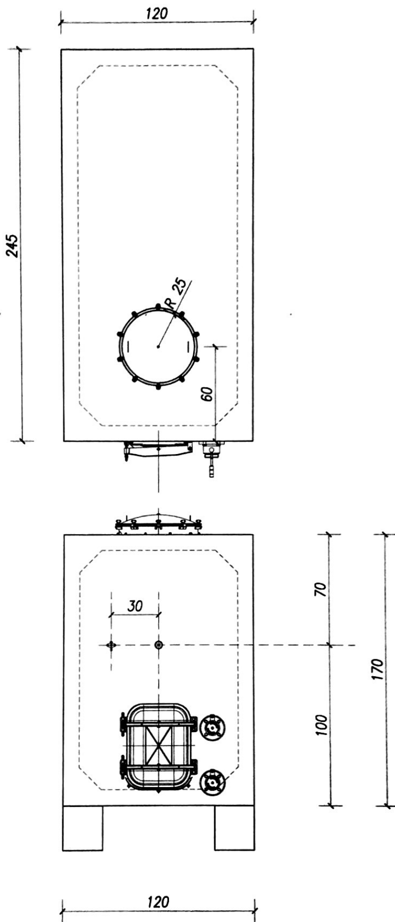
N°6 CISTERNE CON CAPACITA' 30hl
