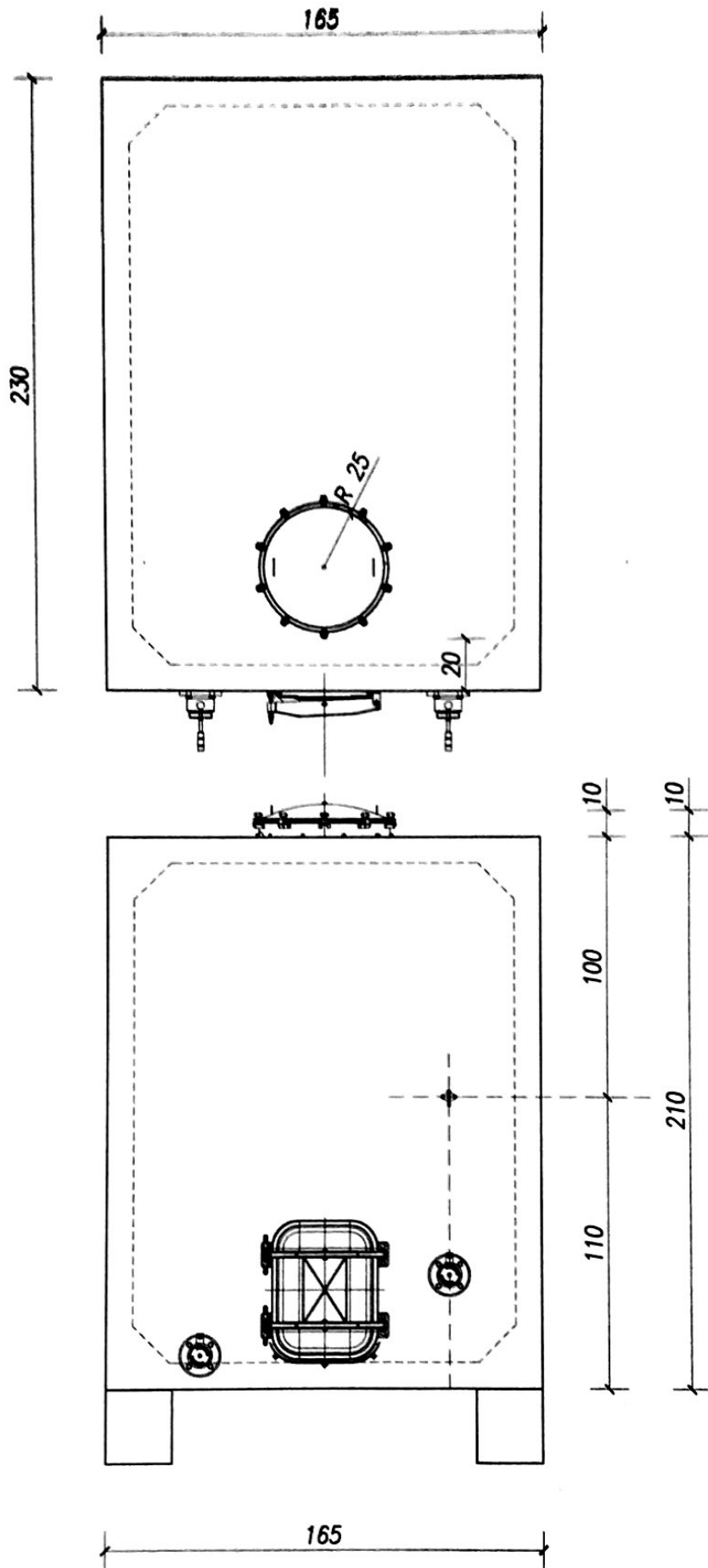
N°1 CISTERNE CON CAPACITA' 53hl CON VERNICE
