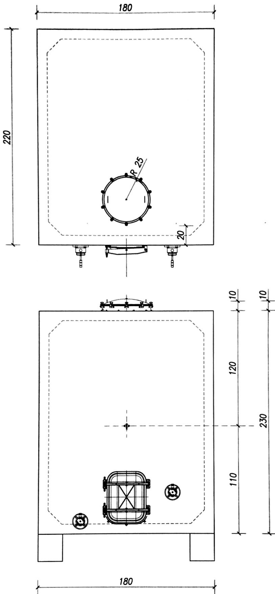
N°2 CISTERNE CON CAPACITA' 62hl CON VERNICE
