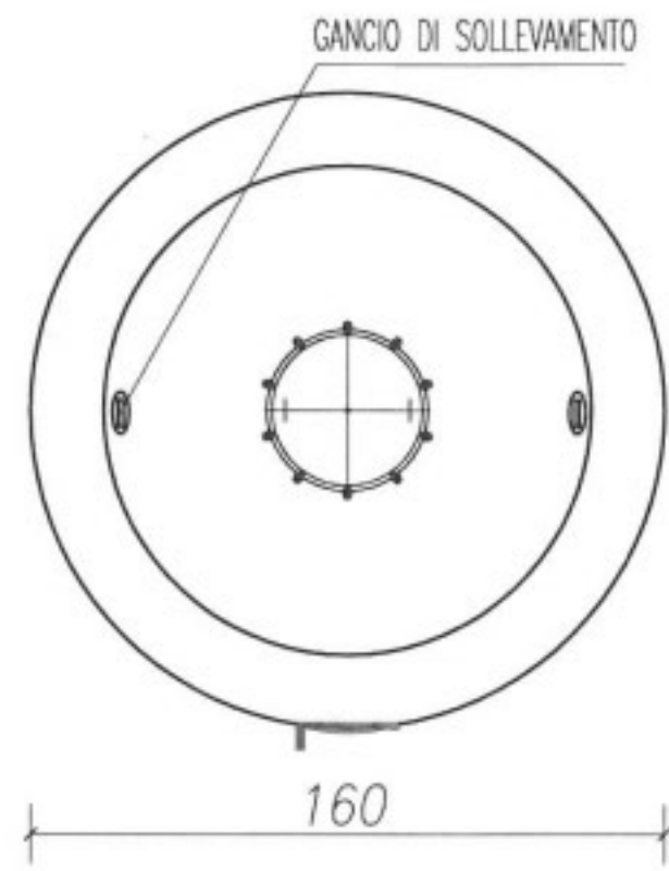
VISTA IN PIANTA
